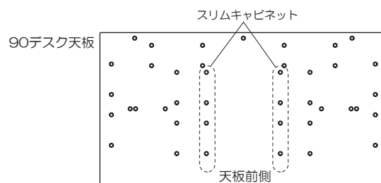
使用する天板裏のネジ穴位置
